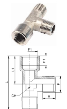
PEMMT: RACOR "TE" LATERAL HEMBRA MxMxH CÓNICO
