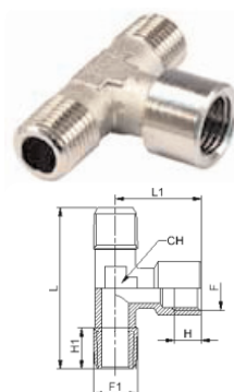
PEMNT: RACOR "TE" CENTRAL HEMBRA MxHxM CÓNICO
